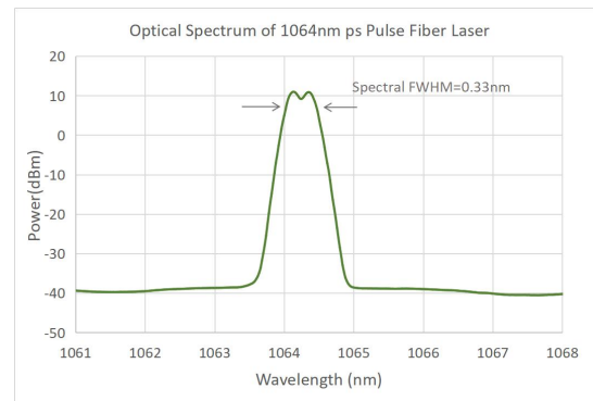
1064nm光谱
