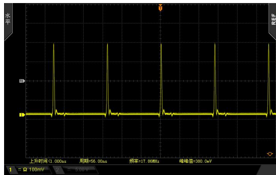
脉冲序列
