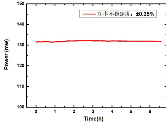
功率稳定
