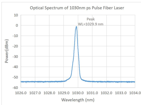
1030nm光谱
